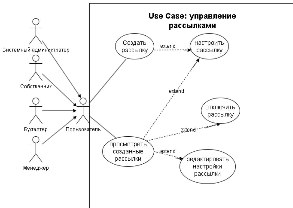
рисунок 1. Диаграмма Use Case для веб-приложения FinSmart
